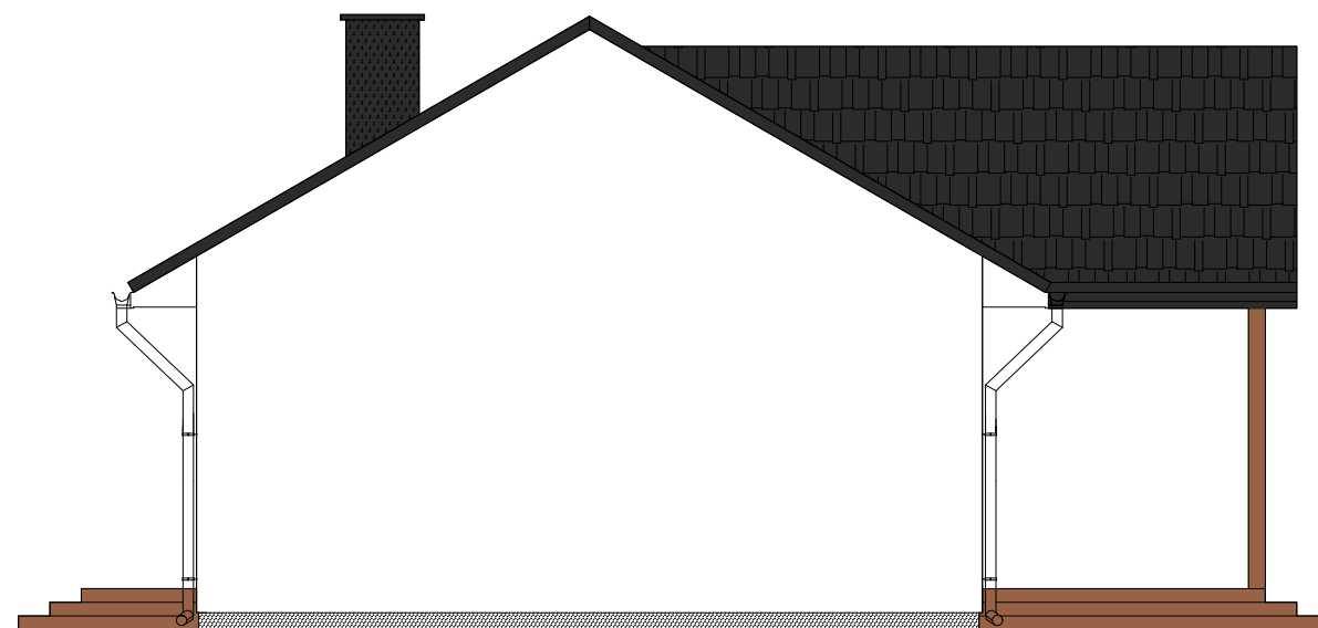
ELEWACJA ZACHODNIA
